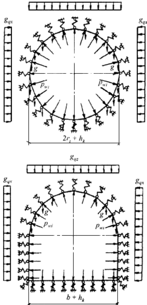
Рисунок А.1 - Расчетные схемы обделок туннелей
